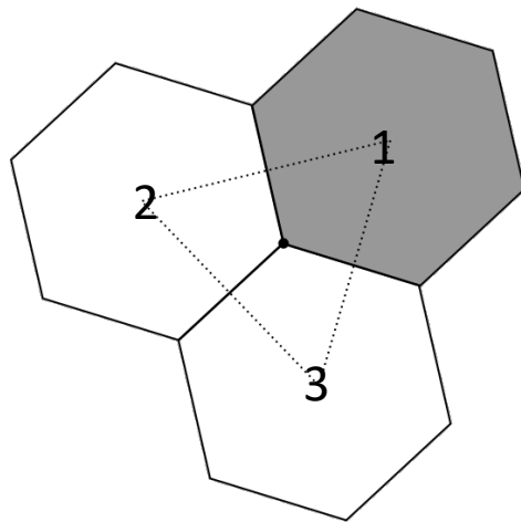
cellsOnVertex(:,V)
